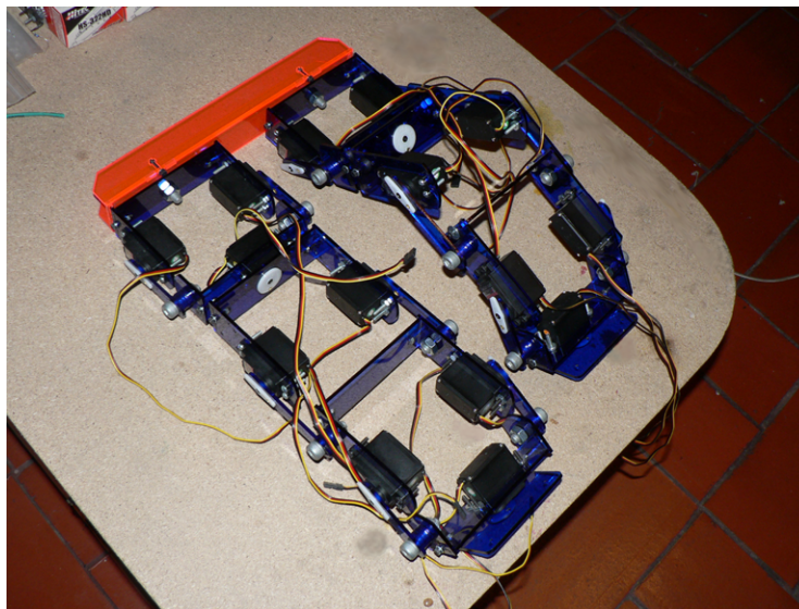
Figura 12. Estructura robótica bípida completamente ensamblada.
