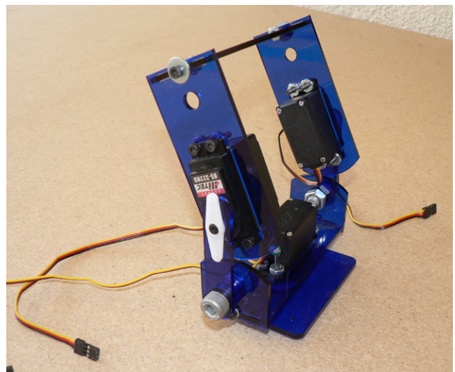
Figura 10. Estructura final ensamblada del tobillo.
