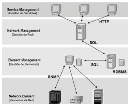
Figura 4. Diagrama estructura lógica [2].
