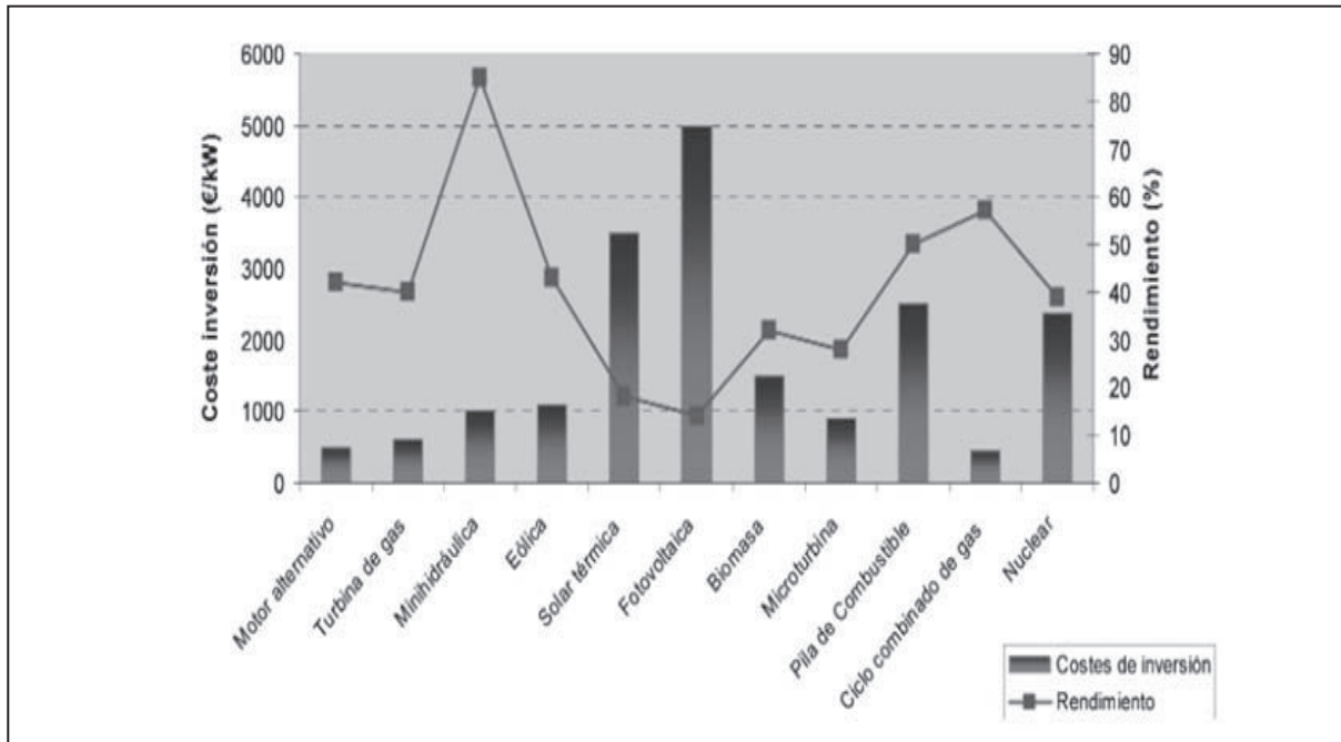
Fig. 2. Comparación de costos de inversión y rendimientos eléctricos para las diferentes tecnologías de generación.
