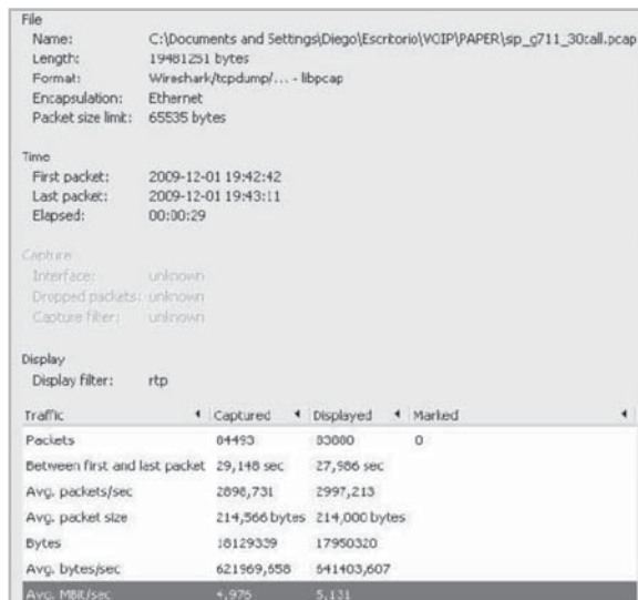
Figura 7. Resumen SIP, G.711, 30 llamadas.
