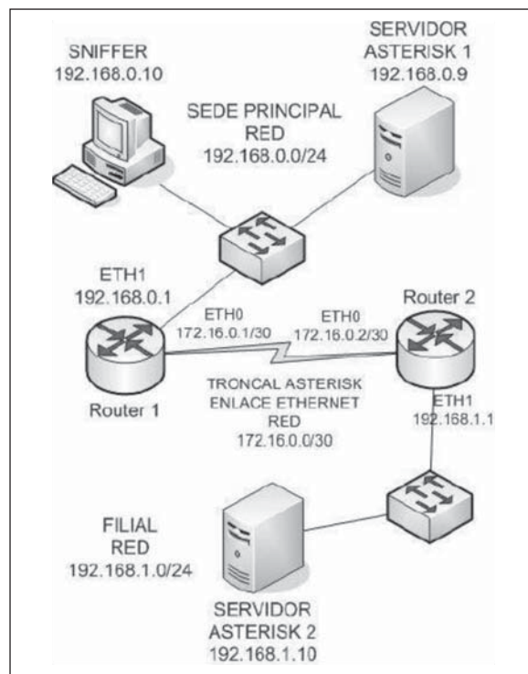
Figura 2. Mapa de red VoIP.
