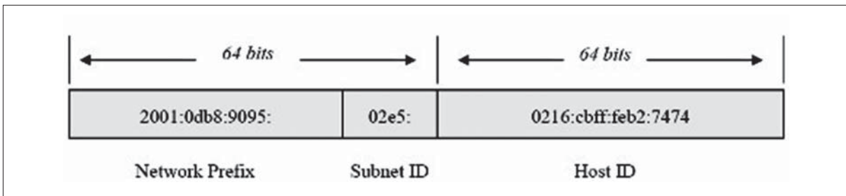
Figura 6. Dirección IPv6 con prefijo de 64 bits
