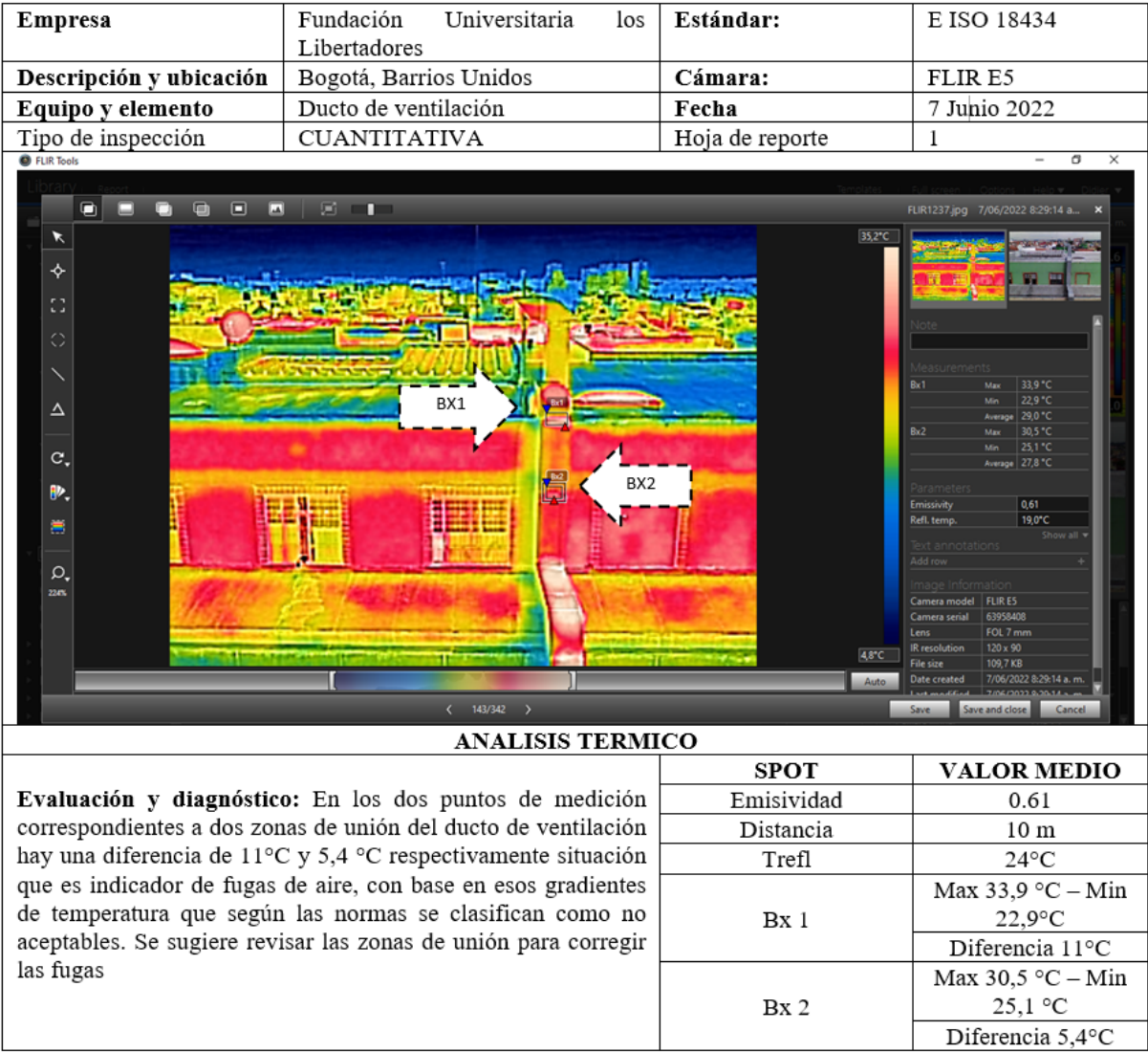
Figura 5. Superficie exterior y el techo de la sede Bolívar Fuente: Autores.
