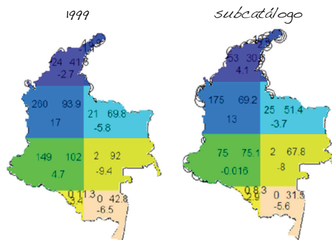
Figura 8. \chi^2 basada en el conteo de cuadrantes, 1999 y subcatálogo
