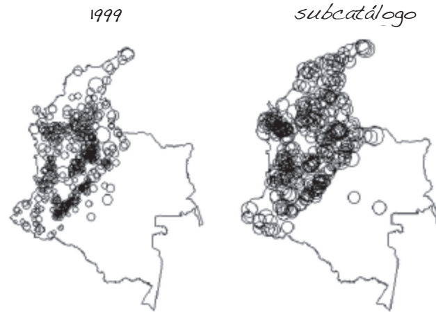
Figura 7. Ubicación de eventos sísmicos, 1999 y subcatálogo
