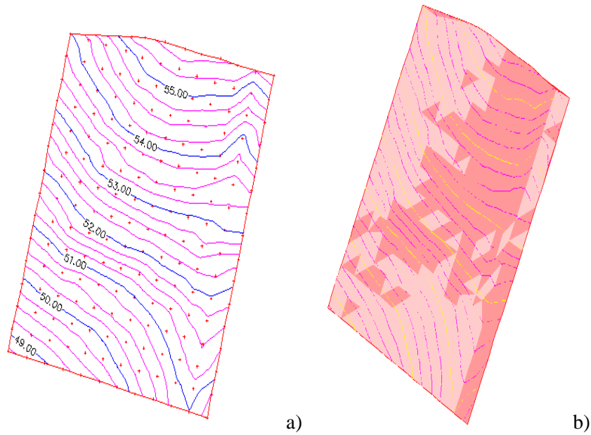
Figura 3. a) Curvas de nivel para la red de levantamiento cada 10 m del terreno; b) vista en 3D
