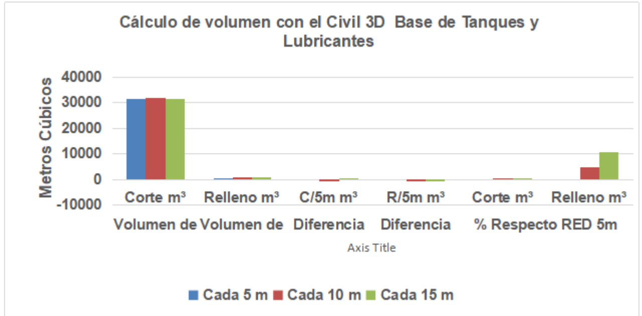
Figura 6. Comparación de los volúmenes obtenidos para diferentes redes del levantamiento
