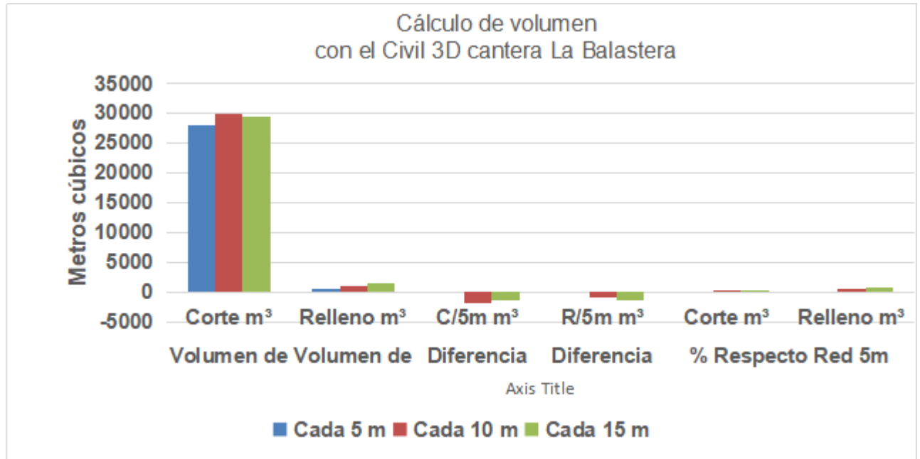
Figura 7. Comparación de los volúmenes obtenidos para diferentes redes del levantamiento
