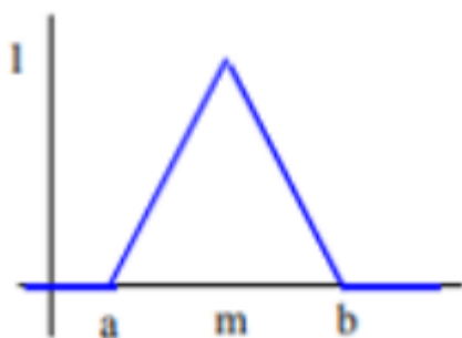
Figura 3: Función lambda.
