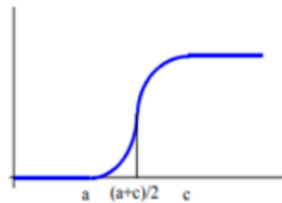
Figura 4: Función S.
