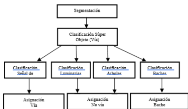
Figura 8: Flujo de clasificación.
