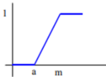
Figura 2: Función gamma.
