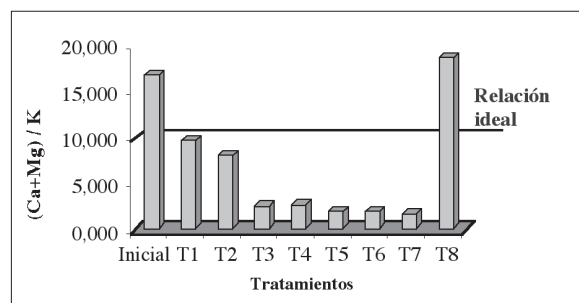
Figura. 12 a. Relación Mg/K entre tratamientos. b. Relación (Ca+Mg)/K entretratamientos. T1 (testigo), T2 (EM), T3 (compost + EM), T4 (mulch + EM), T5 (gallinaza), T6 (fertilización química), T7 (abonos orgánicos + EM), T8 (abonos orgánicos + EM + fertilización química).
