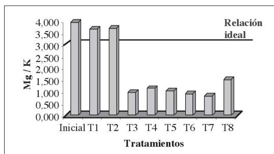
Figura. 12 a. Relación Mg/K entre tratamientos. b. Relación (Ca+Mg)/K entretratamientos. T1 (testigo), T2 (EM), T3 (compost + EM), T4 (mulch + EM), T5 (gallinaza), T6 (fertilización química), T7 (abonos orgánicos + EM), T8 (abonos orgánicos + EM + fertilización química).
