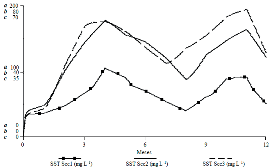
Figura 3. Modelación de los SST en las secciones 1, 2, y 3. a. SST Sec1 (mg L -1 ). b. SST Sec2 (mg L -1 ), c. SST Sec3 (mg L -1 )
