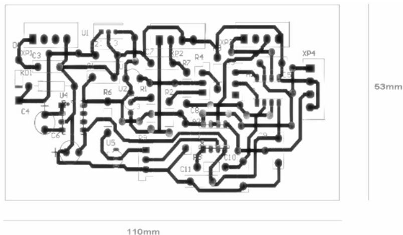
Figura 3. Esquema PCB de la tarjeta acondicionadora.
