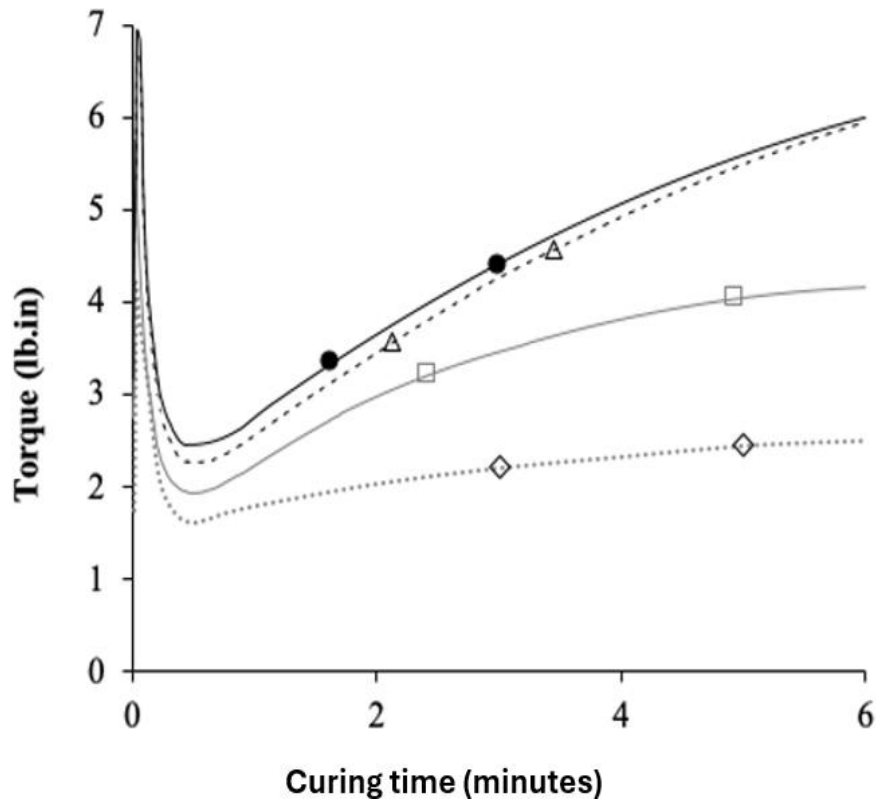
Figure 2. Rheometric curves: —●—NR/0MDTAG --△- -NR/10MDTAG — □—NR/20MDTAG --◇--NR/30MDTAG
