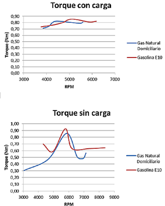
Figura 9. Gráfica Torque vs RPM.
