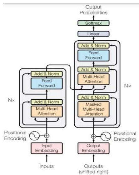
Figura 2-Arquitectura del modelo Transformador [17]
