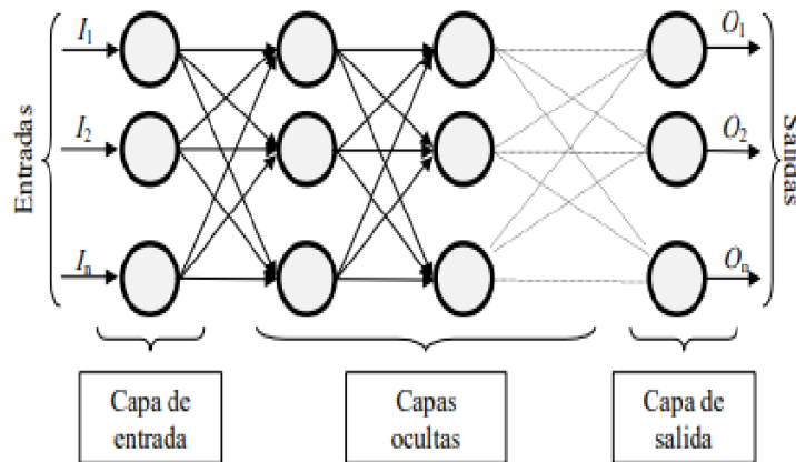
Figura 1. Esquema de una red neuronal tomado de [10]
