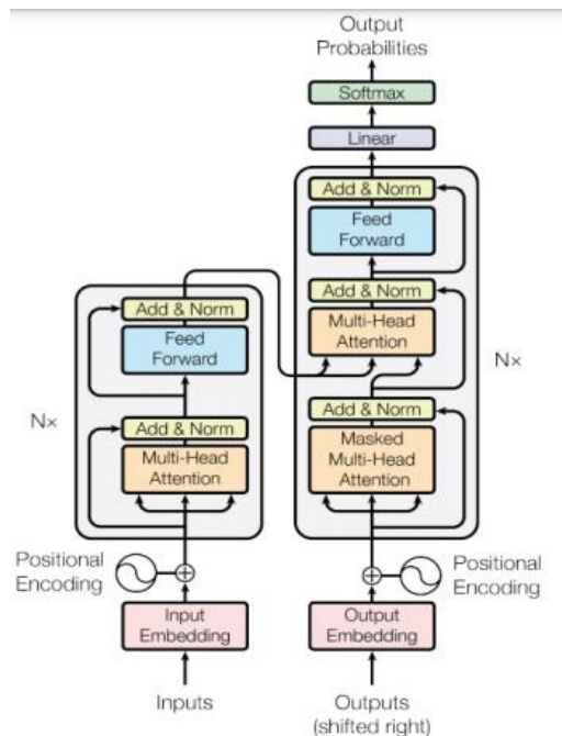
Figura 2-Arquitectura del modelo Transformador [17]
