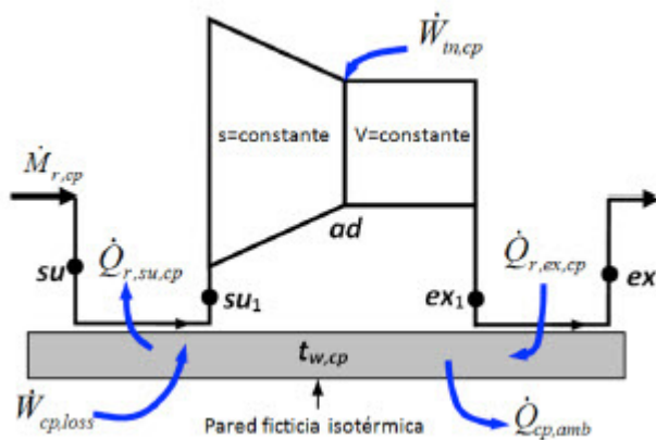
Figura 4. Principio de la modelación del compresor [14].
