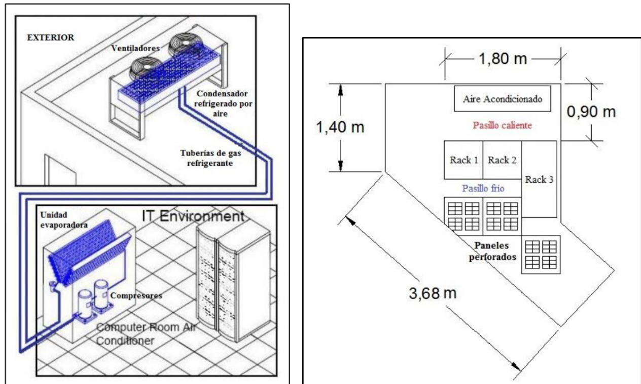
Figura. 11 a) Componentes del sistema de climatización. b) Ubicación de paneles de salida [39].
