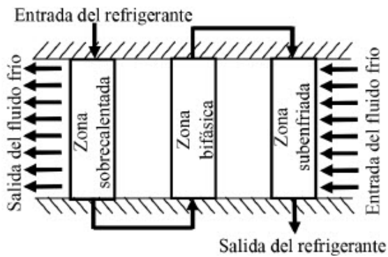
Figura 5. Principio de la modelación del condensador [14].
