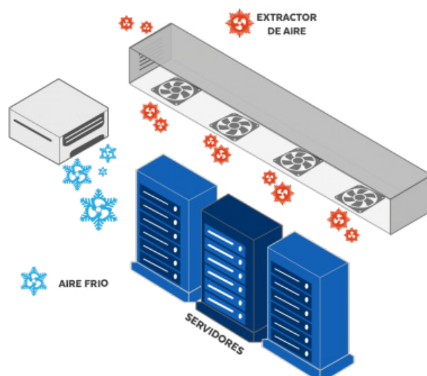
Figura 3. Unidad de Climatización centro de datos [8].
