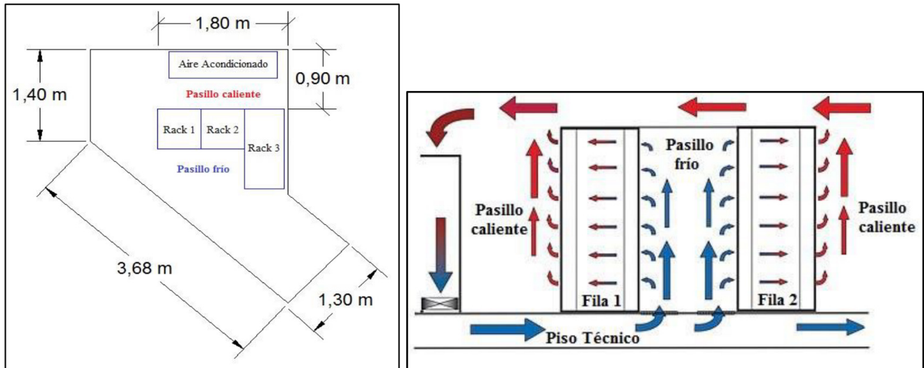
Figura 10. a) Ubicación del equipo de aire acondicionado dentro de centro de datos. b) Distribución de flujo de aire en el centro de datos. Ejemplo 1 [39].
