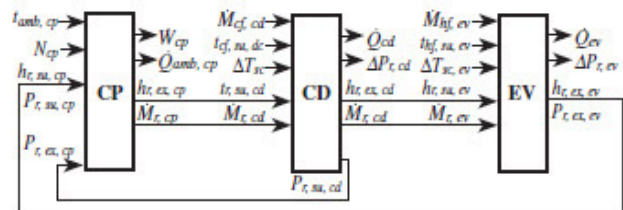
Figura 7. Principio del modelado del sistema de refrigeración [14].
