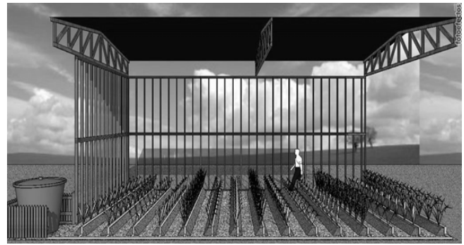
Figura 6: Diseño de la distribución en planta en línea de la huerta urbana en Sierra Morena, Bogotá D.C. Vista Frontal. Fuente: elaboración propia
