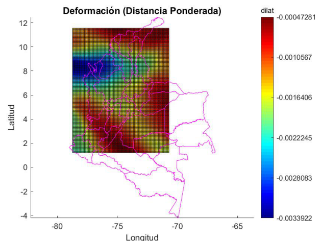
Figura 5. Mapa de dilatación elaborado en Matlab con el código Grinstrain Fuente: elaboración
