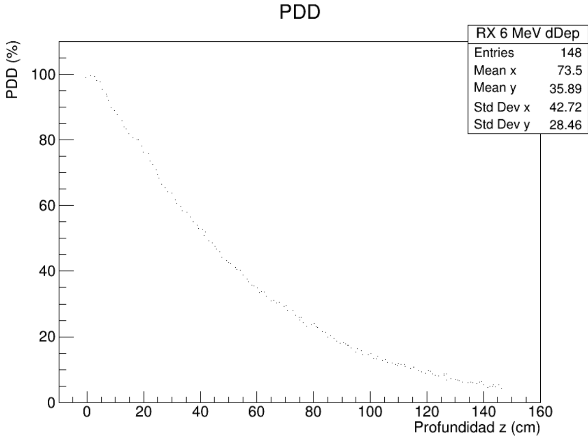
Figura 7: PDD del cubo de agua simulado
