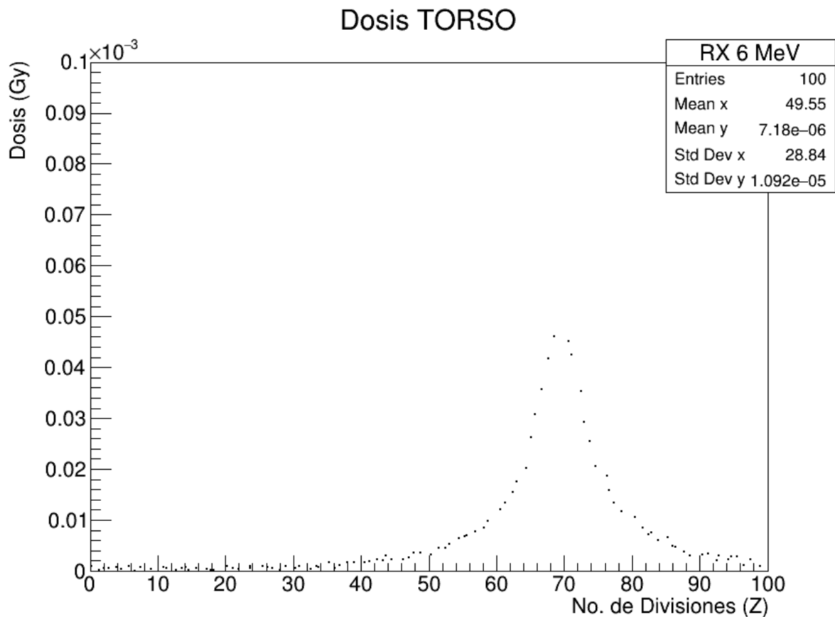
Figura 6: Gráfica correspondiente a la dosis depositada en el isocentro.
