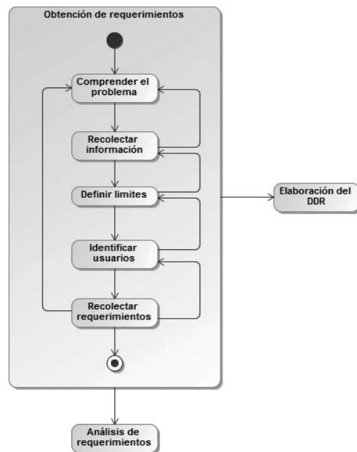
Figura 2. El proceso de obtención de requerimientos
