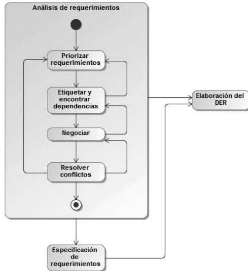
Figura 3. El proceso de análisis de requerimientos.
