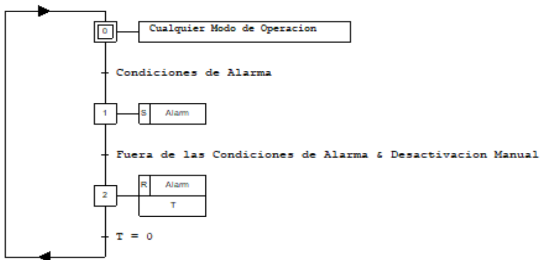
Figure 12. Alarm Grafcet.
