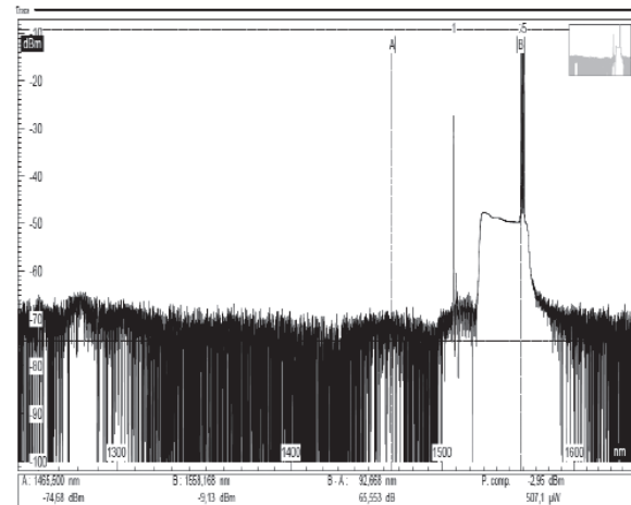
Gráfica 1. Salida de analizador DWDM.
