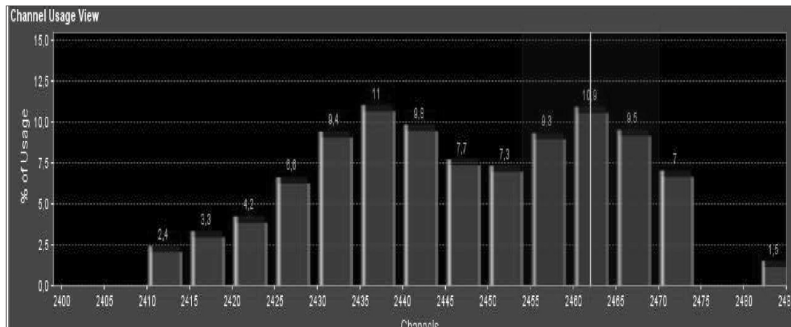
Figura 3. Medición de canales en 2,4 GHz con analizador de espectro para los nodos de la red inalámbrica
