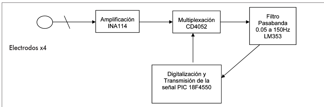
Figura 6. Diagrama de bloques hardware del sistema
