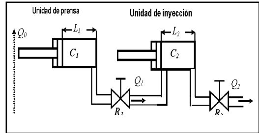
Figura 7. Sistema hidráulico (prensa e inyección)
