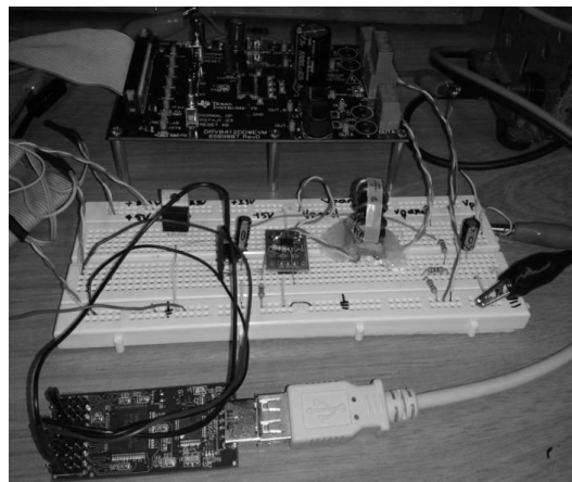
Figura 7. Hardware implementado para pruebas del algoritmo.
